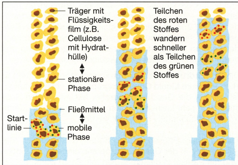
Abb. 1: Trennung eines Substanzgemisches durch Papier- oder Dünnschichtchromatographie
