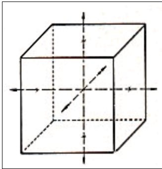
Abb. 1: Würfel
