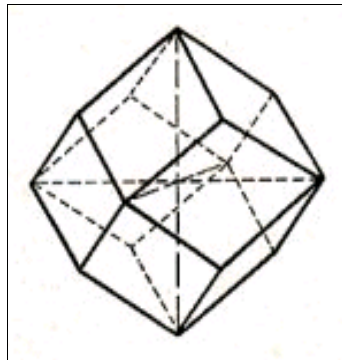
Abb. 5: Rhombendodekaeder
