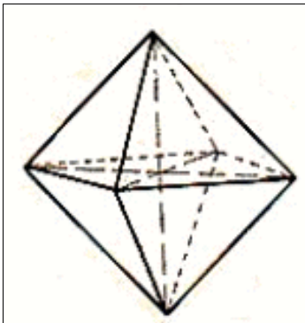
Abb. 4: Oktaeder
