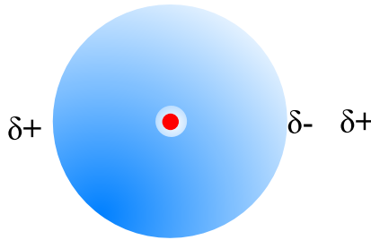
Atom mit asymmetrischer Ladungsverteilung
