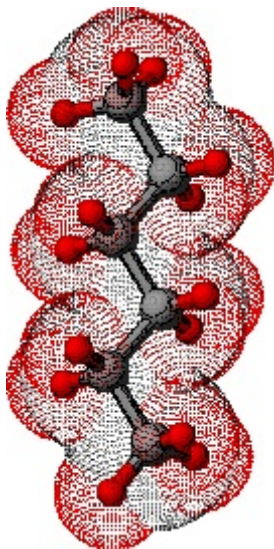
n-Hexan-Molekül mit Oberfläche und gleichmäßiger Ladungsverteilung
