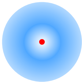
Atom mit kugelsymmetrischer Ladungsverteilung
