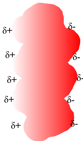
Oberfläche des n-Hexan-Moleküls mit ungleichmäßiger Ladungsverteilung
