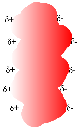
Oberfläche des n-Hexan-Moleküls mit ungleichmäßiger Ladungsverteilung
