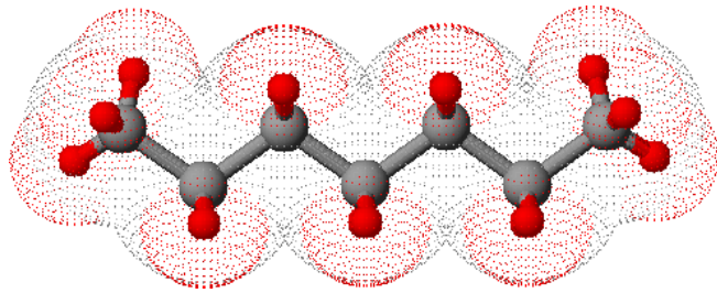
n-Heptan
